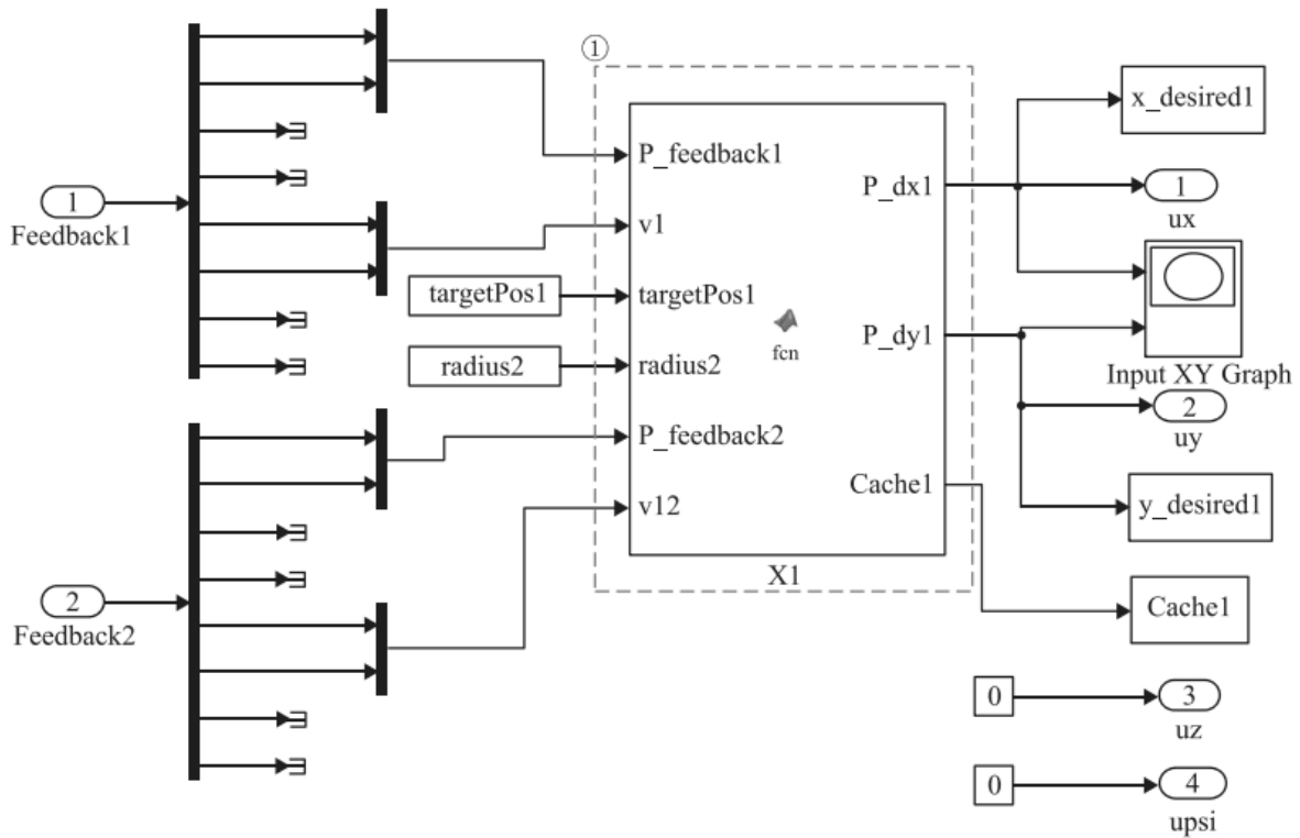
图 8.39 各通道控制输入
