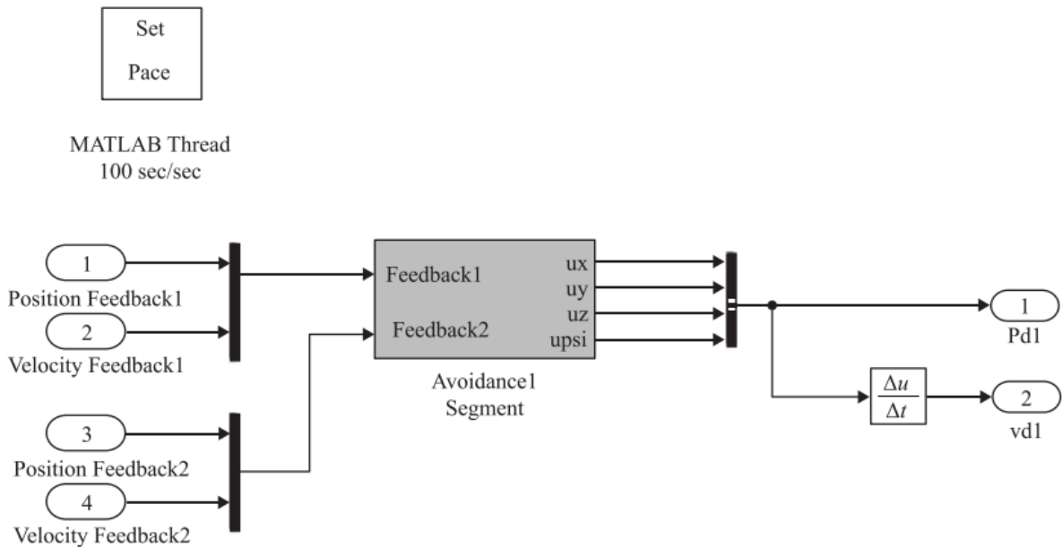
图 8.38 控制输入模块
