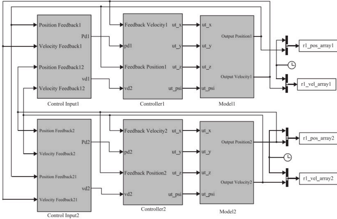
图 8.37 整体模块，Simulink 模型详见“e5\5.4\sim1.0\5_4_Avoidance_Segment.slx”
