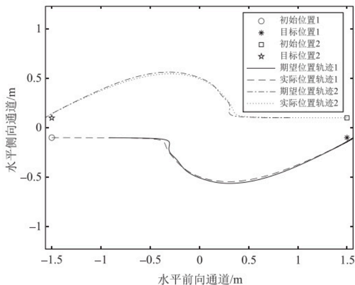
图 8.40 期望位置轨迹和实际位置轨迹对比
