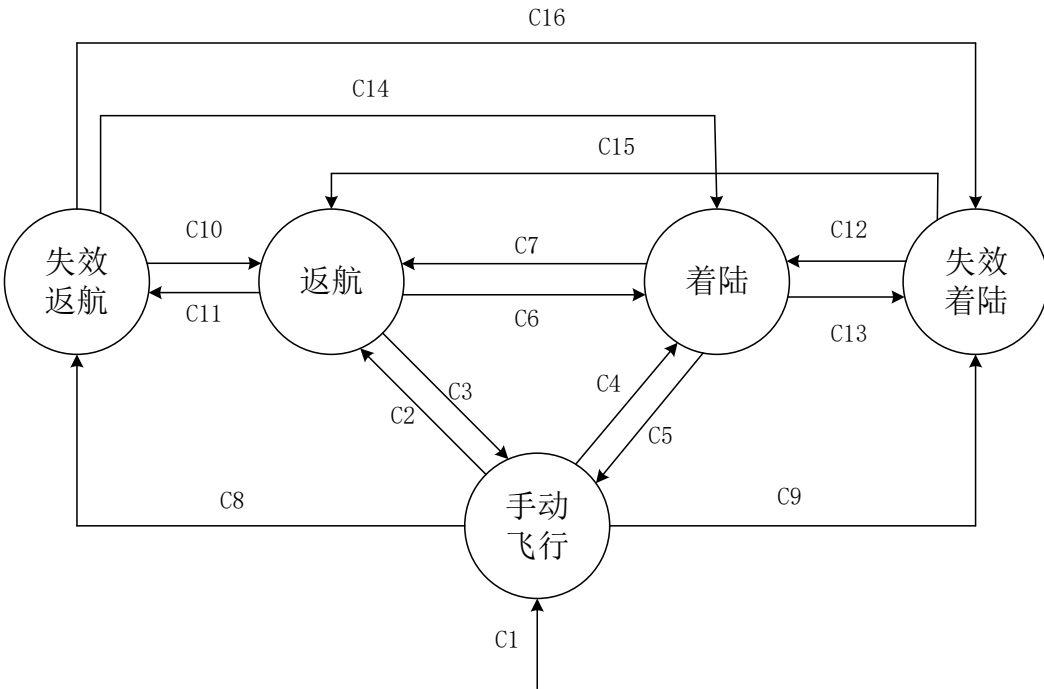
图. 状态机
